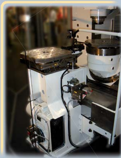
Palettenwechsler
